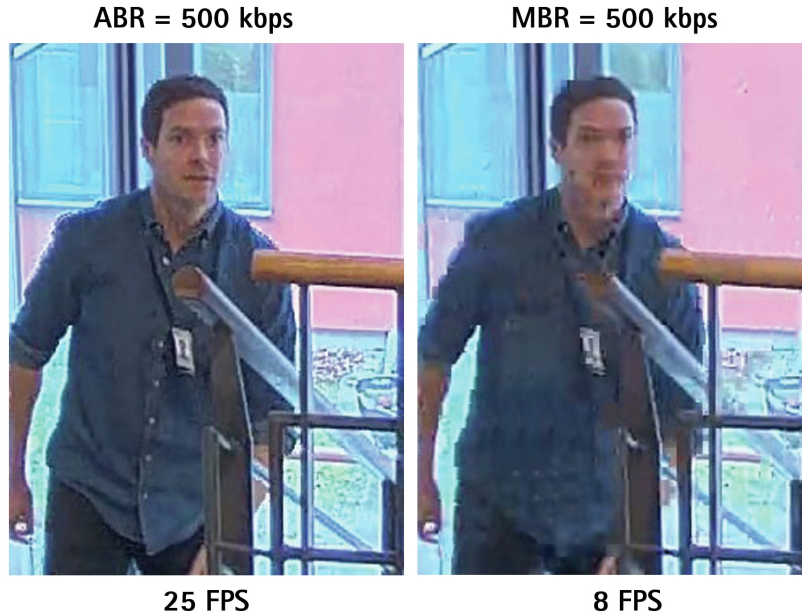
Figure 1. 움직임이 많은 대용량 장면의 비디오에서 잘라낸 스냅샷. 이미지 품질과 프레임 레이트는 ABR의 경우 훨씬 더 높았습니다. 이 방법을 사용하면 매우 조용한 장면에서 짧은 시간의 움직임이 발생하는 동안 훨씬 더 높은 순간 비트 레이트(약 4000kbps)가 가능하기 때문입니다.
