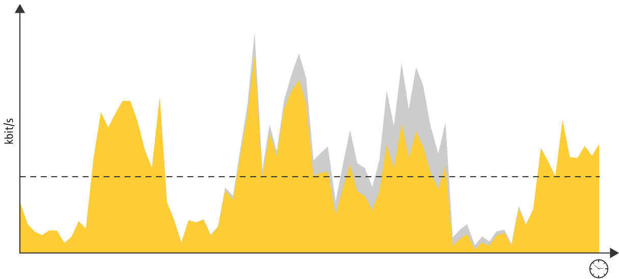
Figure 2. ABR을 사용하면 초기의 유휴 기간의 절약 덕분에 피크 이벤트 발생 시에도 높은 이미지 품질을 유지할 수 있습니다. 설정된 기간 동안 평균화된 비트 레이트 목표를 달성해야 합니다.
