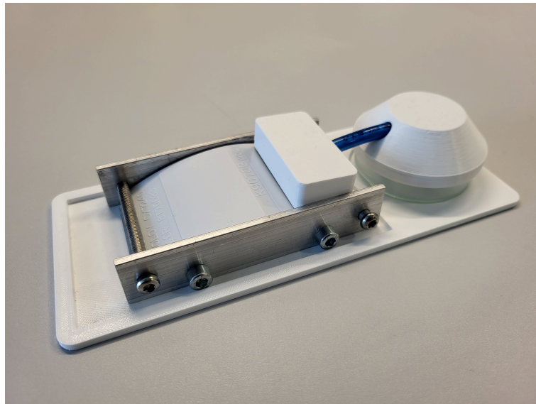
Abbildung 3.1 Einrichtung für Prüfungen zur Beständigkeit gegen umweltbedingte Spannungsrissbildung
