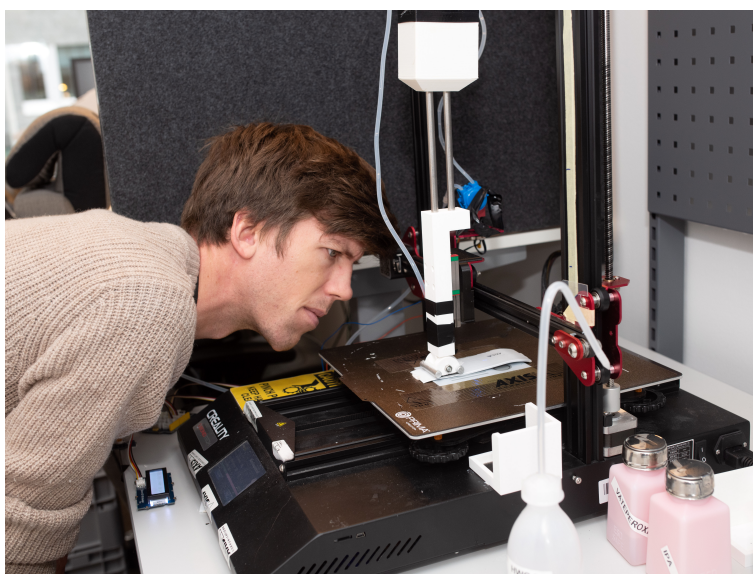
Figura 3.2 Equipos utilizados para la simulación de limpieza. Las muestras se limpiaban con un paño montado en un brazo móvil automático.
