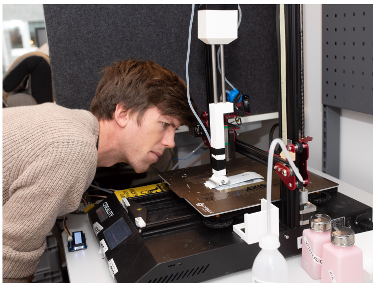
Figure 3.2 Installation pour la simulation de nettoyage. Les échantillons sont essuyés avec un chiffon fixé à un bras mobile automatique.
