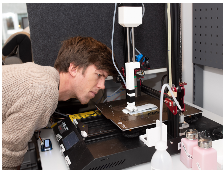
Figura 3.2 La simulazione di pulizia. I campioni vengono strofinati con un panno fissato su un braccio mobile automatico.
