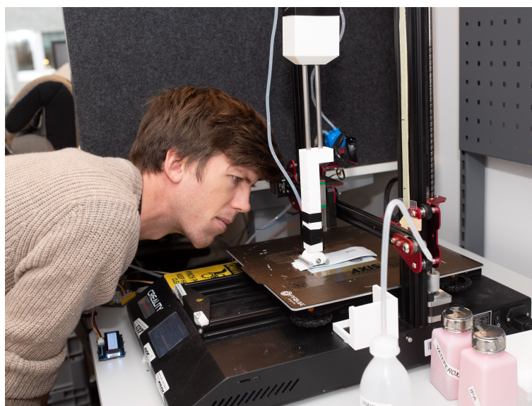
図 3.2 クリーニングシミュレーションのセットアップ。自動可動アームに取り付けられた布で、サンプルを拭き取ります。
