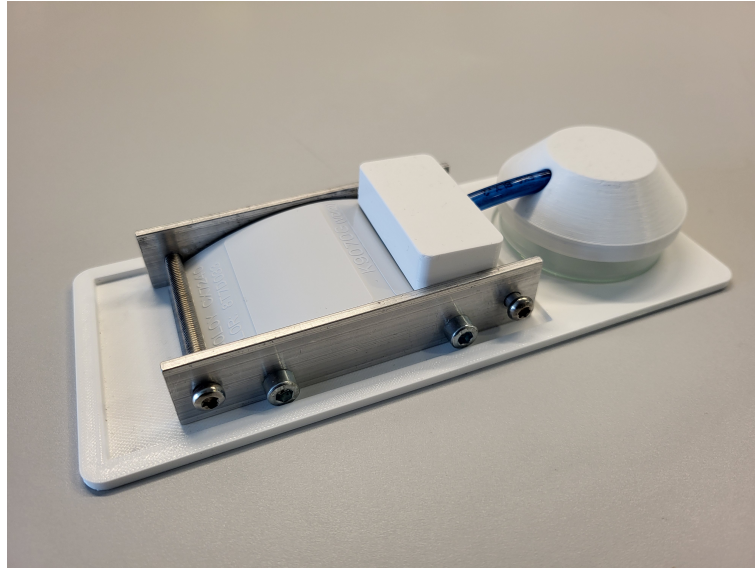
그림 3.1 환경 스트레스 균열 내성 테스트를 위한 설정.
