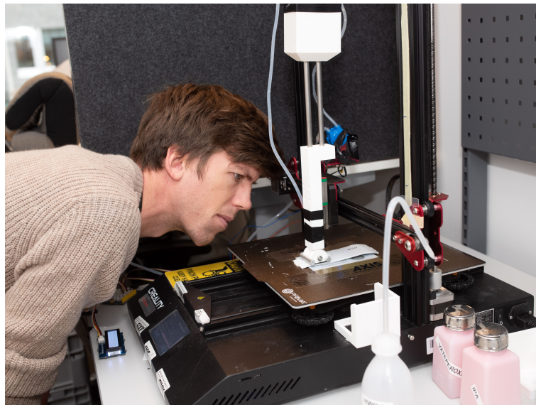
그림 3.2 세척 시뮬레이션을 위한 준비. 샘플은 자동 이동식 암에 장착된 천으로 닦습니다.
