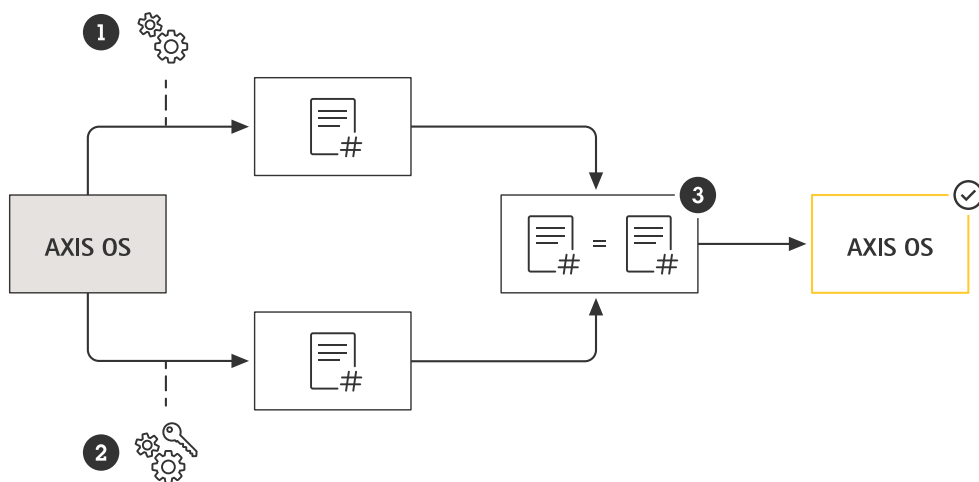
Processus de vérification du système d'exploitation signé.
