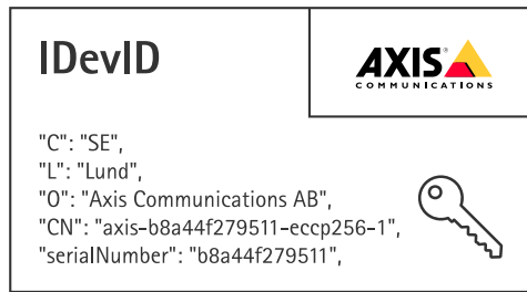
Exemplo de uma ID de dispositivo Axis.
