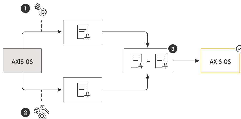
O processo de verificação do SO assinado.
