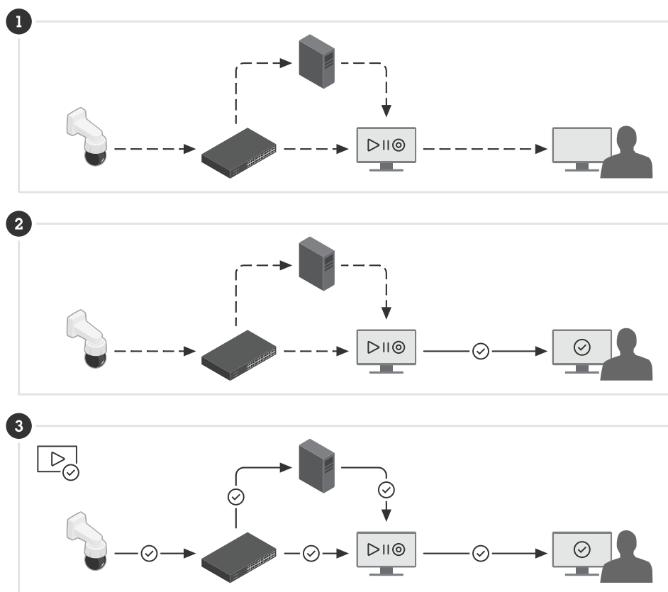
Verificação de autenticidade de vídeo.
