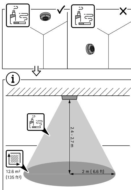
Cobertura de un sensor montado en el techo para detectar el consumo de vapeadores o cigarrillos.
