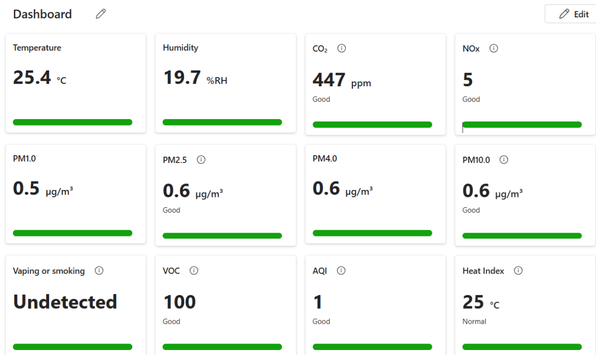
Panel de control que recoge datos de medición en tiempo real de un sensor de calidad del aire Axis.
