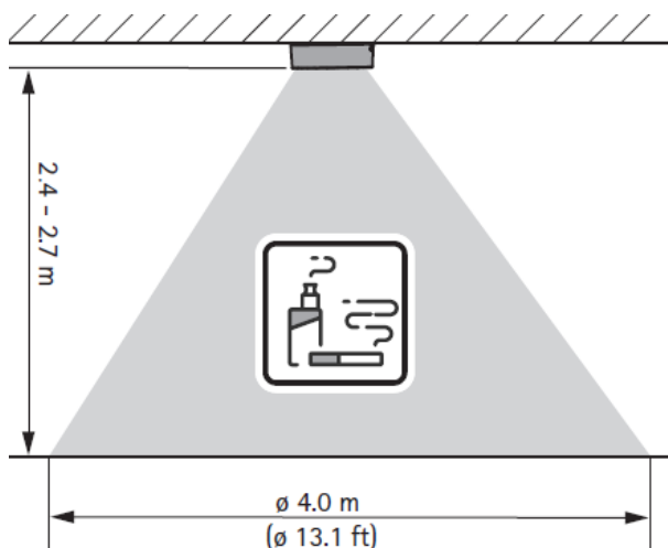
Champ de vision d'un capteur monté au plafond pour la détection du tabagisme ou du vapotage.
