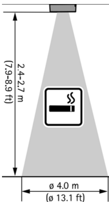
喫煙や電子タバコを検知するための天井に取り付けられたセンサーの範囲。
