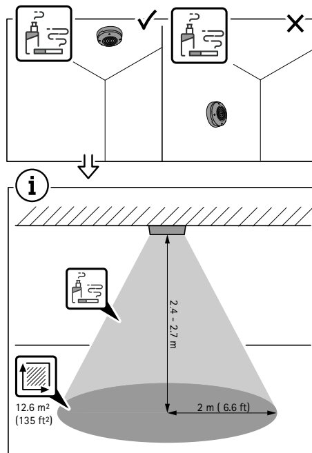
일반 흡연 또는 전자 담배 흡연을 감지하기 위한 천장 장착형 센서의 커버리지.
