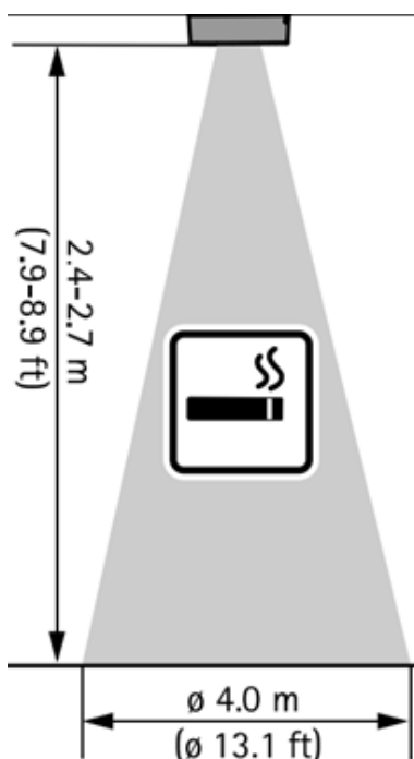
Pokrycie czujnika montowanego na suficie na potrzeby wykrywania palenia tytoniu lub papierosów elektronicznych.
