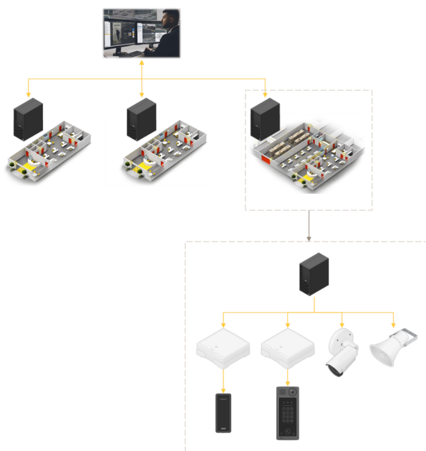
Visão geral do sistema multisite do AXIS Camera Station Secure Entry.
