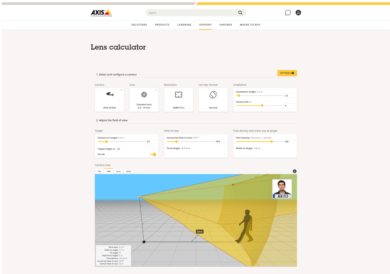
Figura 4.1 Uno screenshot di Lens Calculator.
