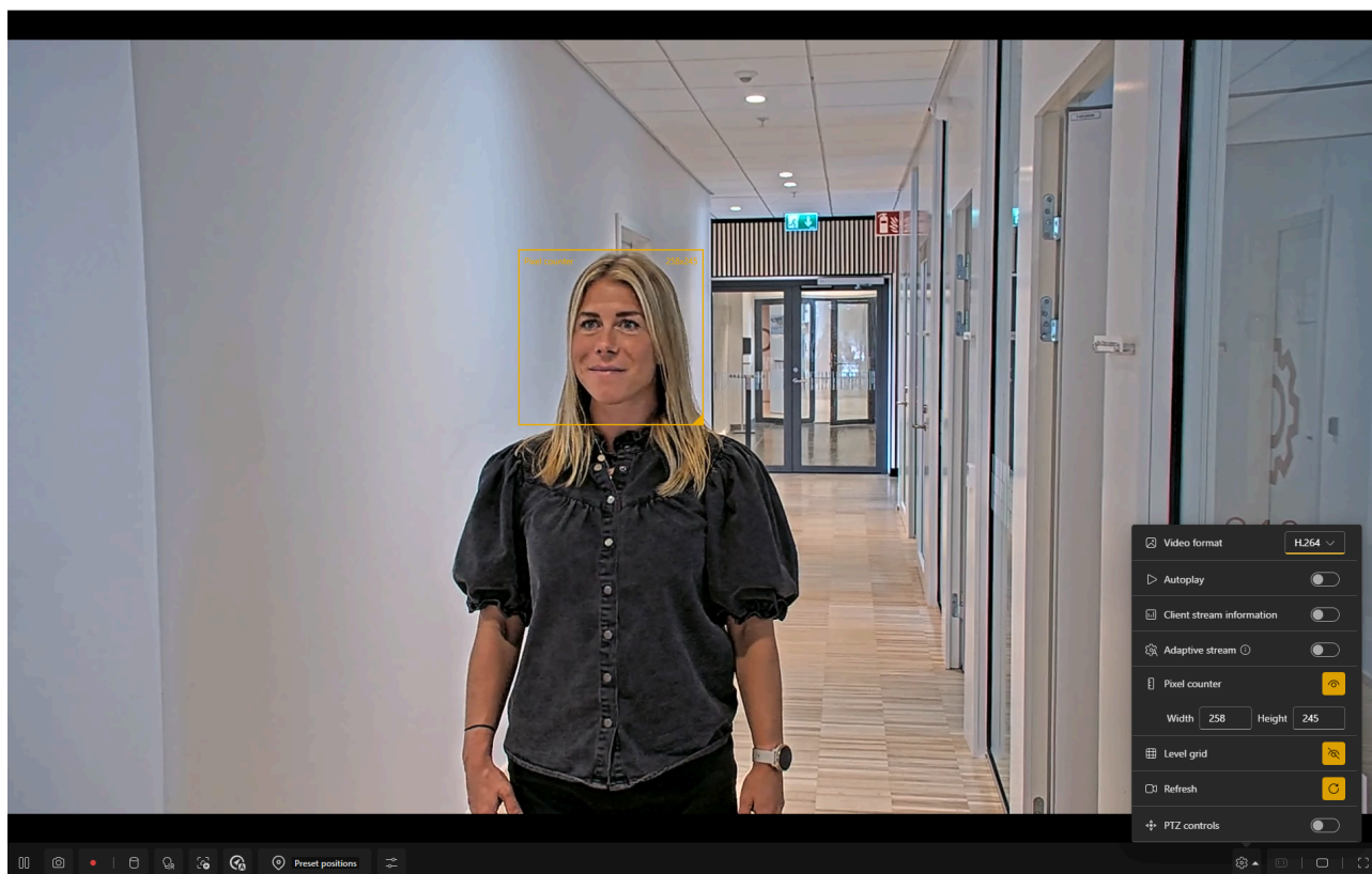
图 4.2 显示了像素计数器的摄像机画面。此工具显示, 边框范围内有258个像素, 这就意味着, 可以达到验证目的 (其要求人脸至少包含80个像素)。
