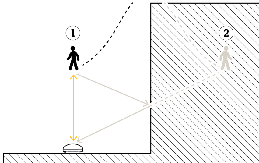
Abbildung 4.2 Bei Wänden oder ähnlichen Objekten in Reichweite des Radars kann es schwierig sein, durch Reflexionen verursachte Falscherfassungen (2) von tatsächlichen Erfassungen (1) zu trennen. In diesem Beispiel könnten Sie das Problem minimieren, indem Sie einen Ausschlussbereich um die Wand herum einrichten.
