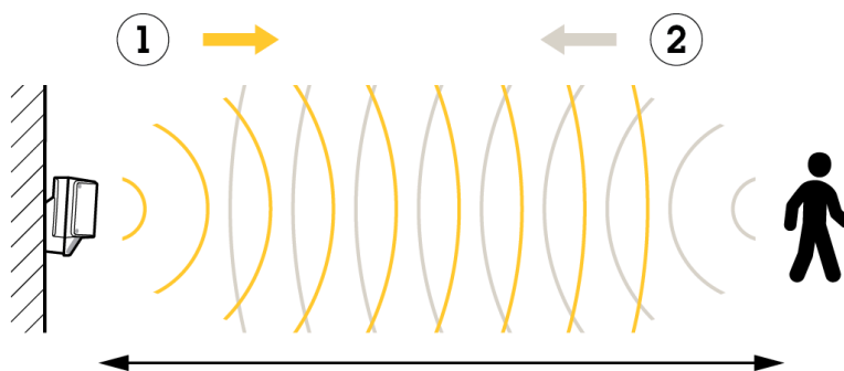
Ilustracja 2.1 Ogólna zasada działania radaru: sygnał (1) emitowany przez radar odbija się (2) od obiektu.
