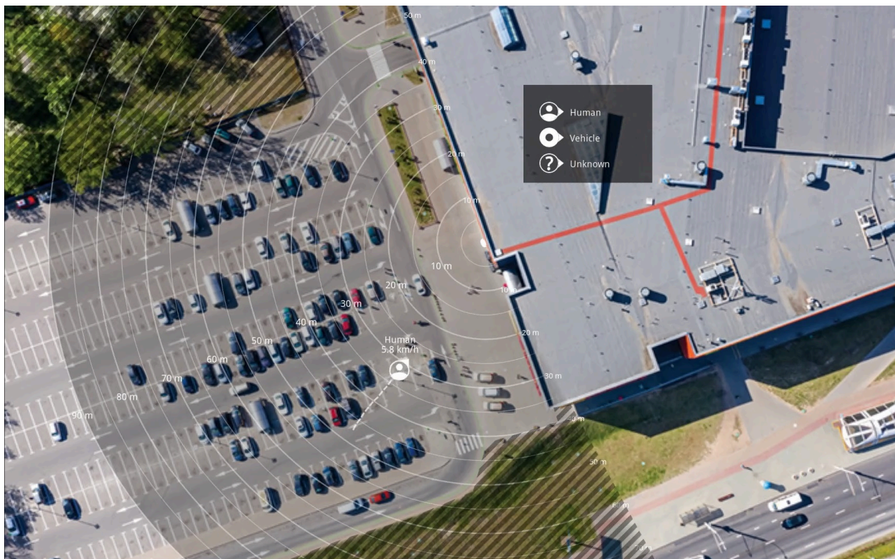
Ilustracja 4.1 Zrzut ekranu interfejsu użytkownika radaru Axis z obrazem referencyjnym sceny.
