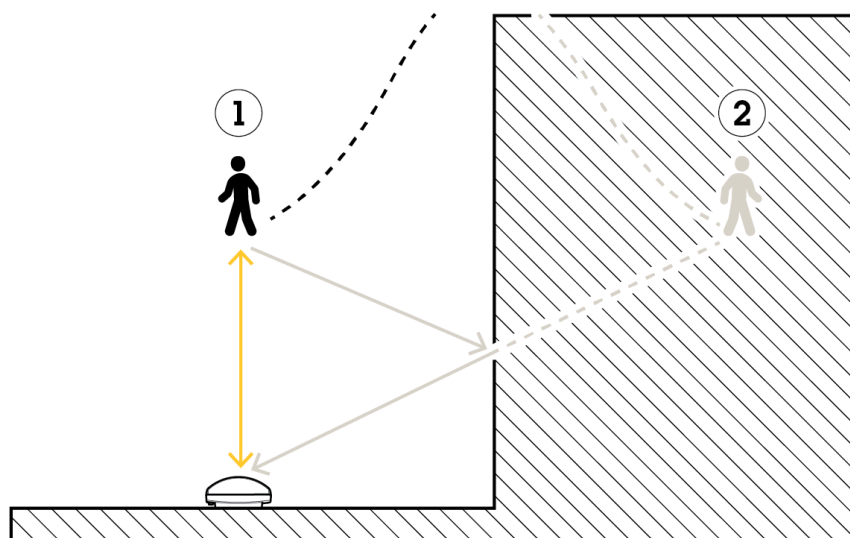
Ilustracja 4.2 W przypadku ścian lub podobnych obiektów znajdujących się w zasięgu radaru fałszywe detekcje (2) spowodowane odbiciem mogą być trudne do odróżnienia od prawdziwych detekcji (1). W tym przykładzie problem można zminimalizować, dodając strefę wykluczenia przy ścianie.
