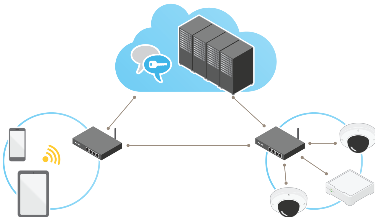
Figura 3.3 Comunicación segura entre iguales entre un cliente y una cámara situados en redes diferentes.
