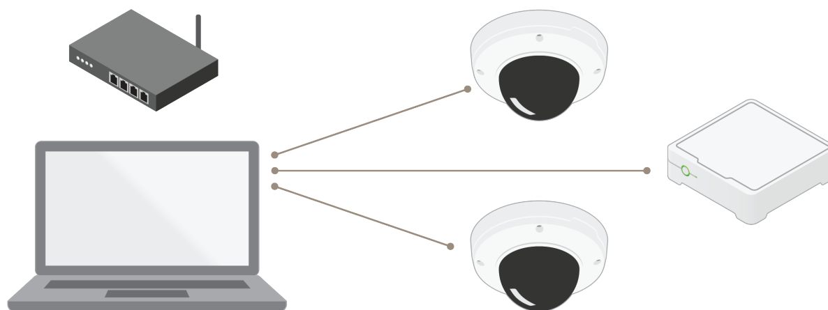
Figura 3.2 Configuración del sistema cuando el cliente y la cámara se encuentran en la misma red.
