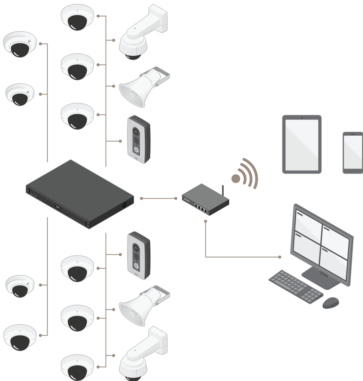
Figura 4.1 Illustrazione di un'installazione con AXIS Camera Station su un sistema basato su AXIS S2016 con switch PoE integrato, 16 dispositivi e client operatore.
