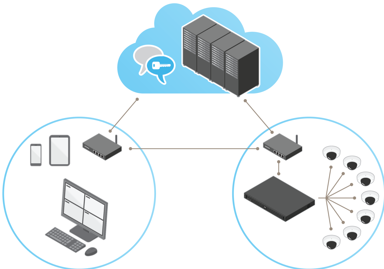
Figura 4.2 Comunicazione protetta, peer-to-peer, tra un client e un server situati su reti diverse e fallback su una comunicazione ritrasmessa.
