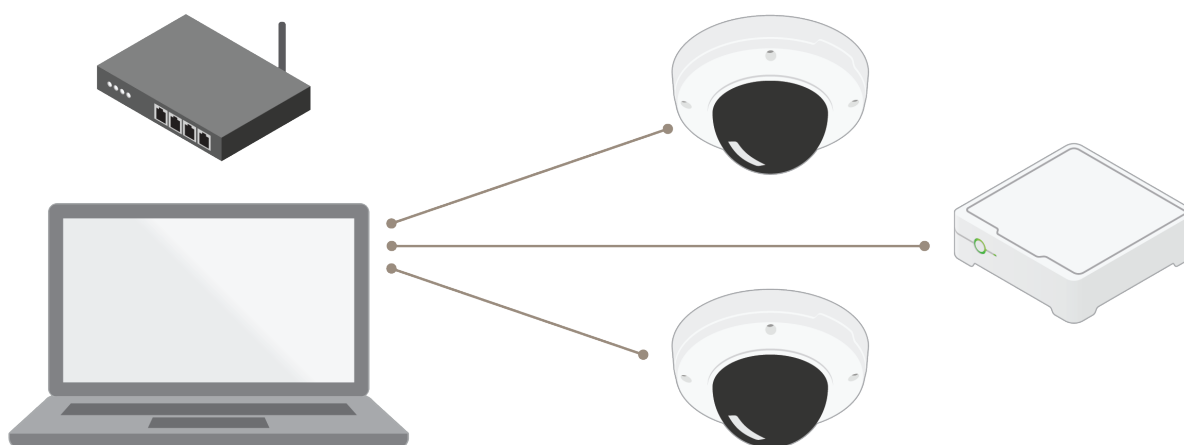
Figura 3.2 Impostazione del sistema quando il client e la telecamera si trovano sulla stessa rete.
