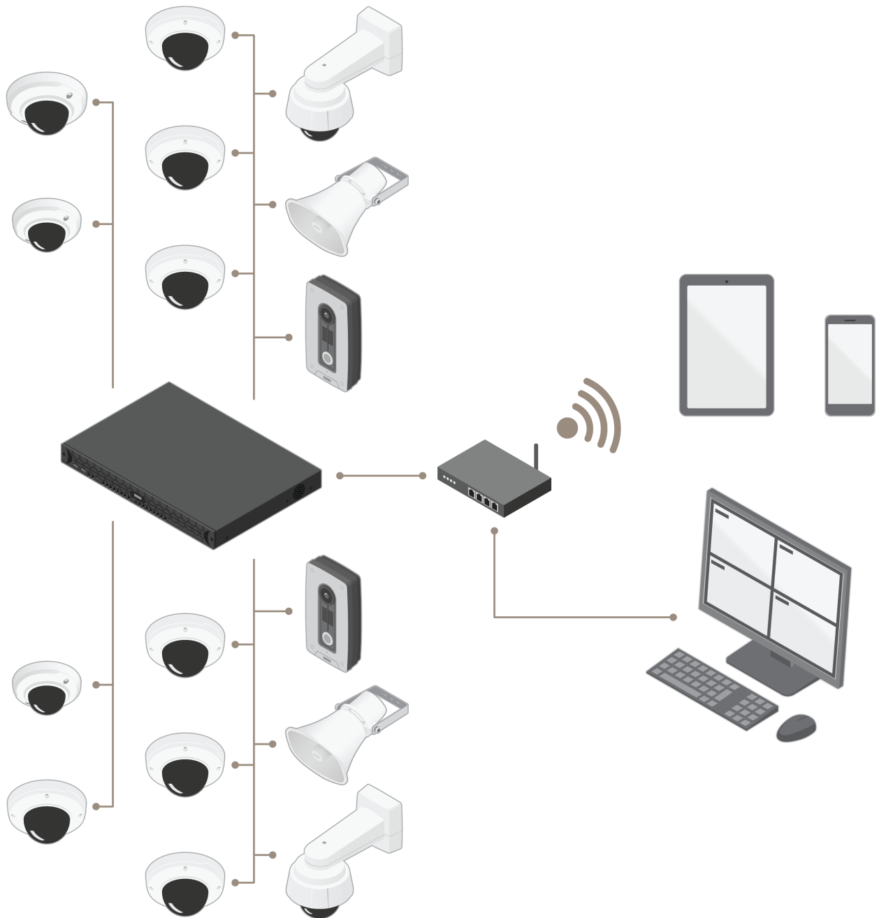
그림 4.1 통합 PoE 스위치, 16개의 장치 및 운영자 클라이언트가 있는 AXIS S2016에서 운영되는 시스템에 AXIS Camera Station을 설치한 그림입니다.
