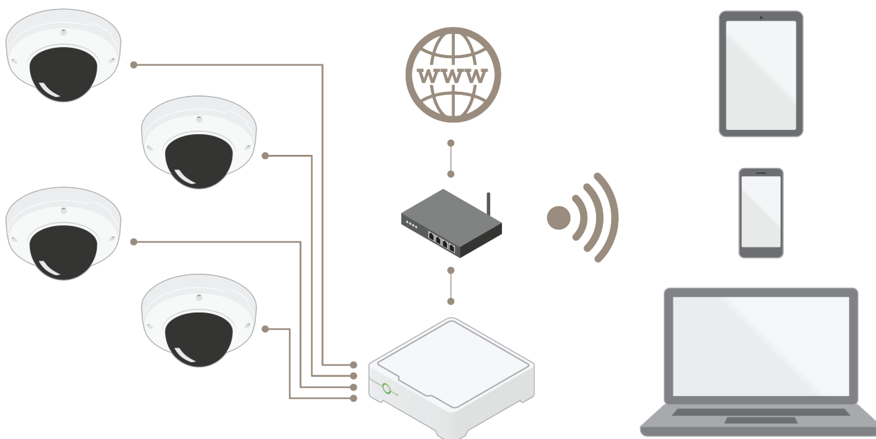
Ilustracja 4.1 Ilustracja systemu AXIS Companion z czterema kamerami, pamięcią masową w postaci kart SD, przełącznikiem PoE, routerem i klientami.
