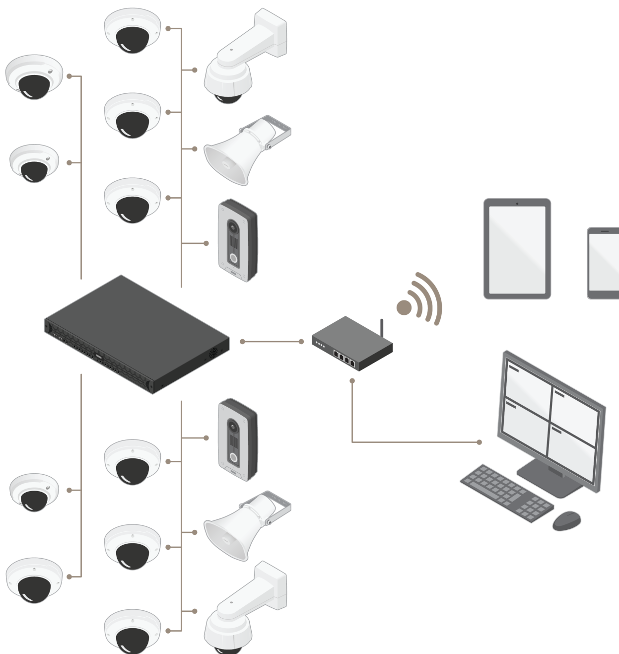
Ilustracja 5.1 Ilustracja instalacji z oprogramowaniem AXIS Camera Station w systemie wykorzystującym rejestrator AXIS S2016 ze zintegrowanym przełącznikiem PoE, 16 urządzeń i klienty operatora.
