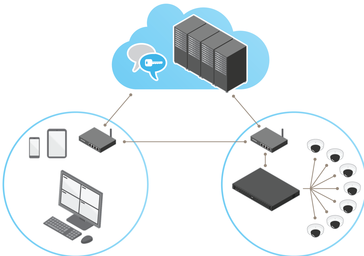
Figura 4.2 Comunicação ponto a ponto segura entre um cliente e um servidor localizados em redes diferentes e fallback para comunicação retransmitida.
