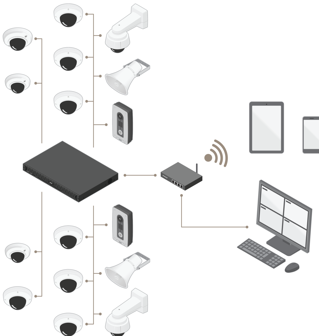
Figura 4.1 Ilustração de uma instalação com o AXIS Camera Station em um sistema executado no AXIS S2016 com switch PoE integrado, 16 dispositivos e clientes operadores.
