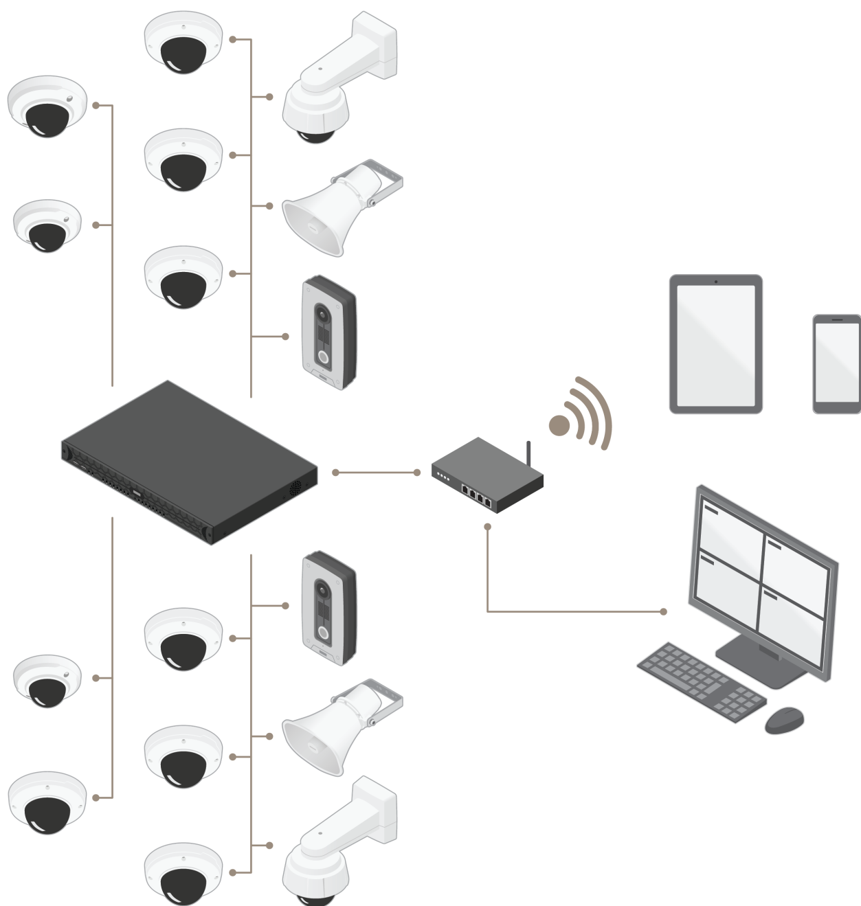
图 5.1 AXIS Camera Station 安装在运行 AXIS S2016 的系统上的示意图，该系统集成了 PoE 交换机、16 台设备和操作员客户端。
