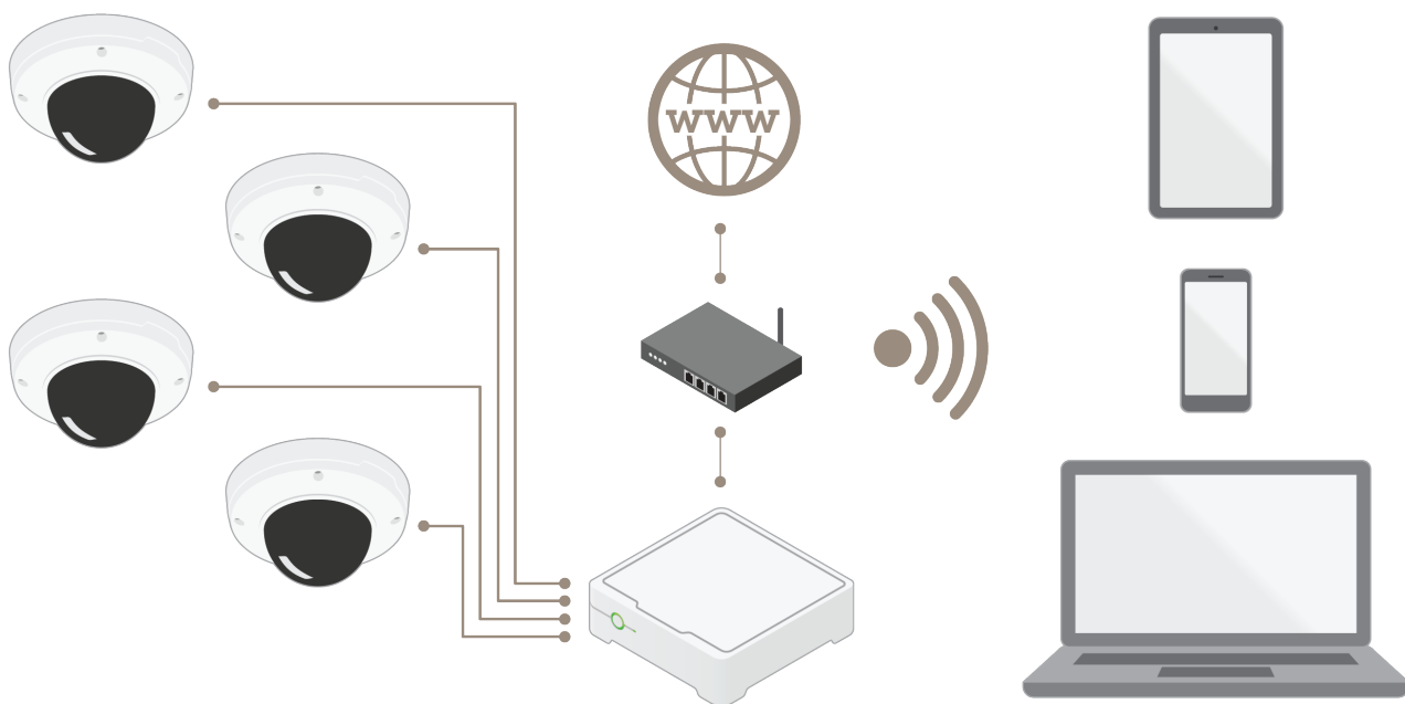
图 4.1 AXIS Companion 系统示意图，包括四台摄像机、SD 卡存储、PoE 交换机、路由器和客户端。
