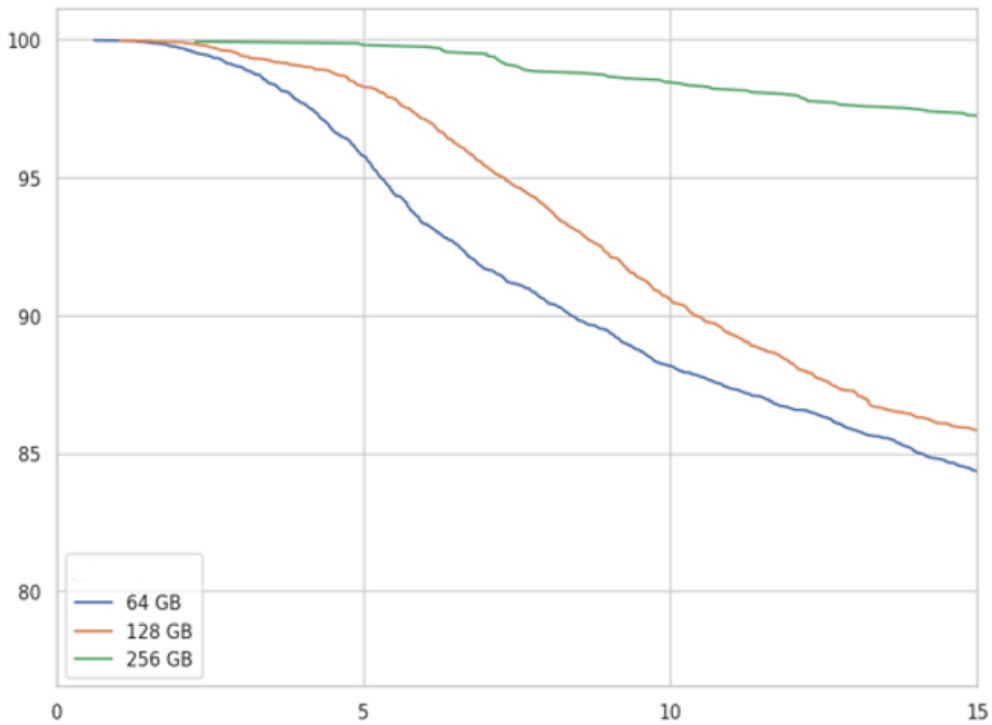
Figure 2. 감시 카드 수명에 대한 누적 백분위수 도표로, 0-15년 후에도 여전히 작동하는 카드의 비율을 보여줍니다. 실제 데이터 및 추정치에 기반한 시뮬레이션.
