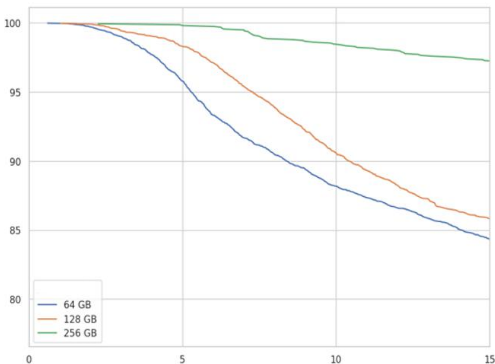
Skumulowany percentylowy wykres żywotności kart do systemów dozoru przedstawiający procent kart działających po 0–15 latach. Symulacja oparta na rzeczywistych danych i szacowaniu.
