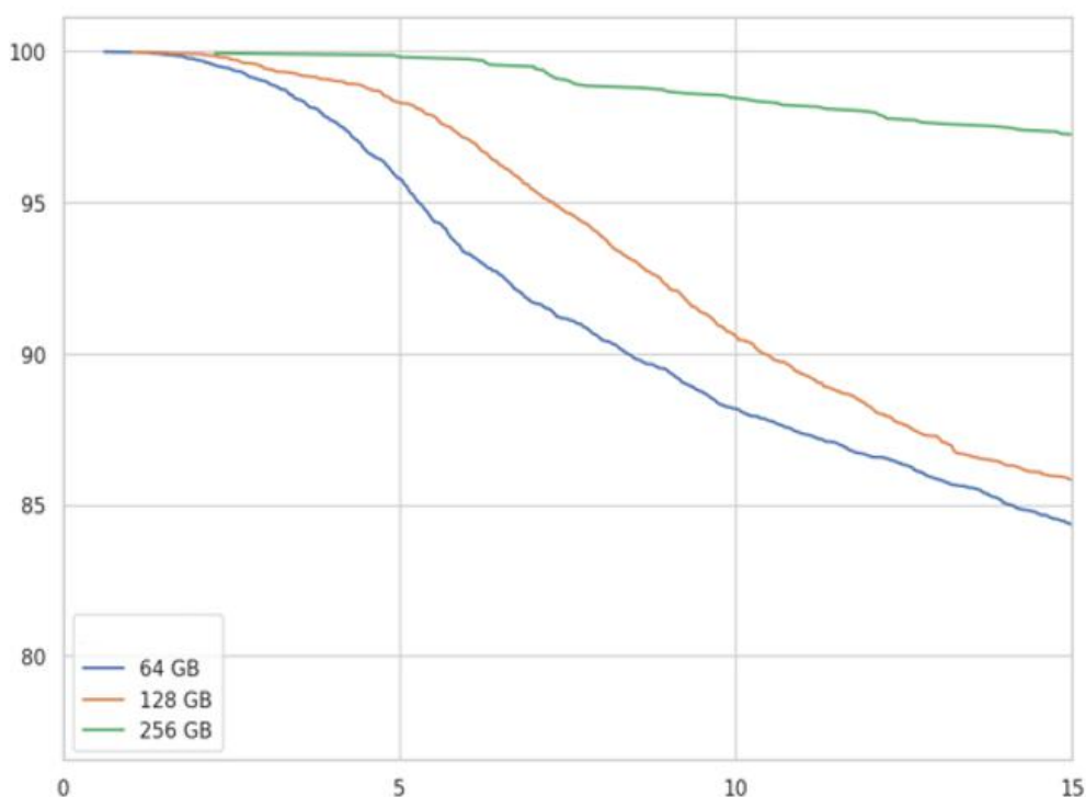
Gráfico de percentis cumulativos da vida útil dos cartões de monitoramento, mostrando quantos por cento dos cartões ainda estão funcionando após 0-15 anos. Simulação baseada em dados reais e estimativas.
