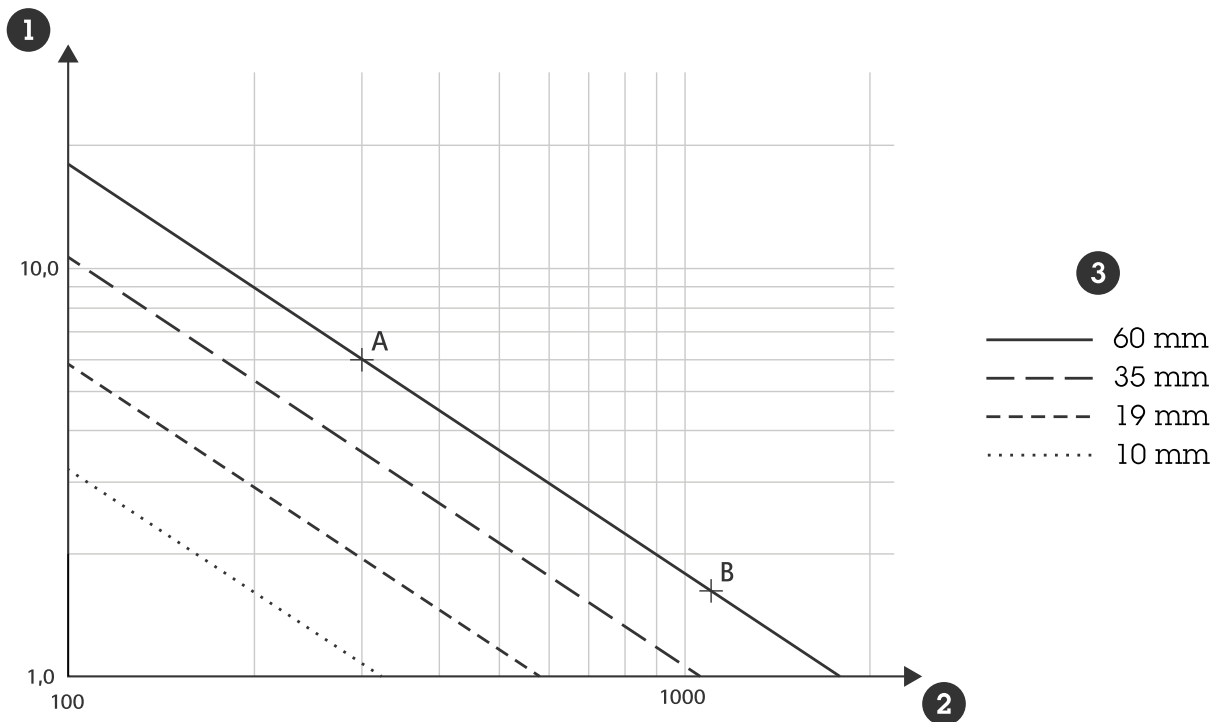
Esempio di un nomogramma per lunghe distanze
